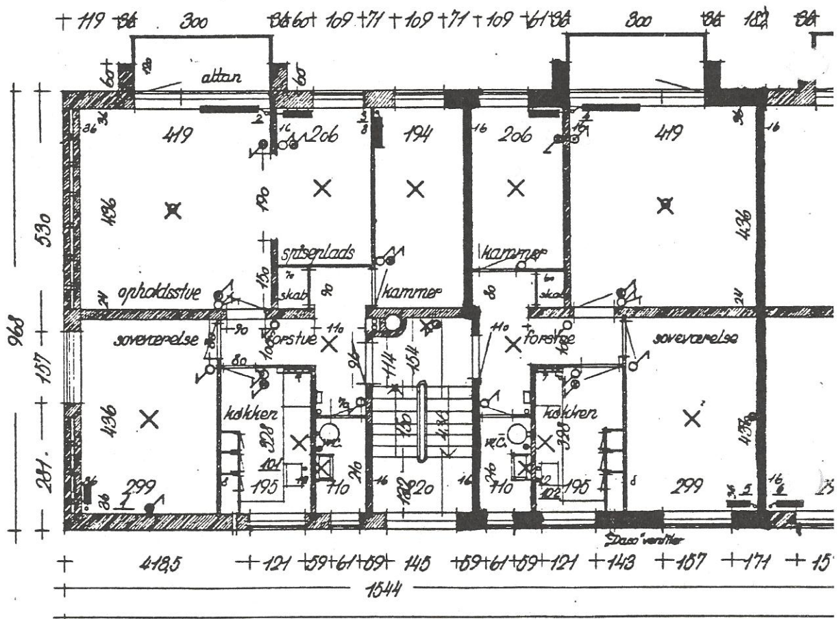
etageplan
