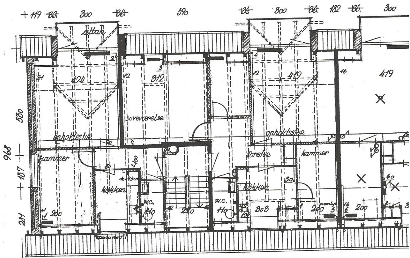
tagplan.
