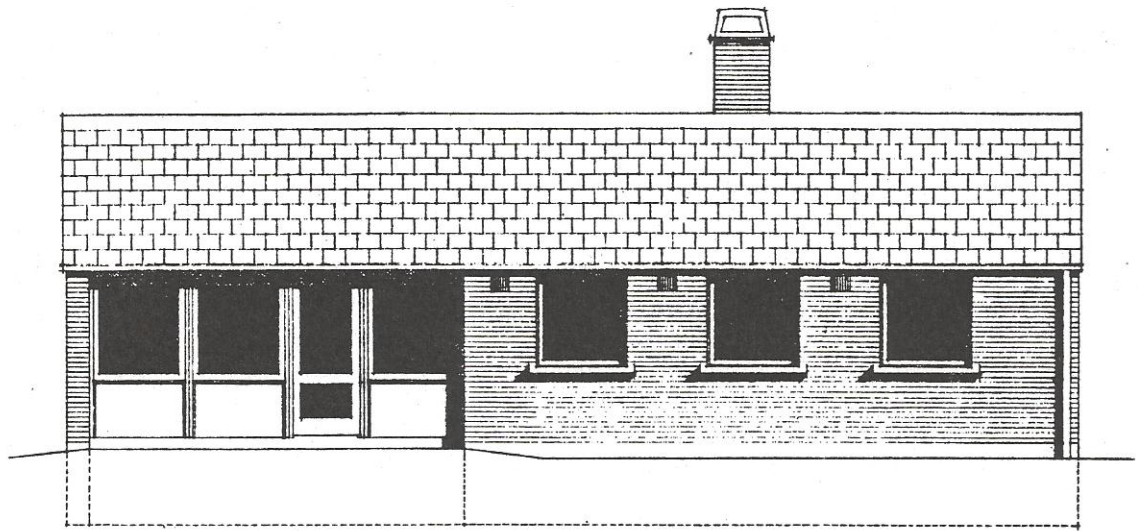
FACADE MOD SYD (VEST)
